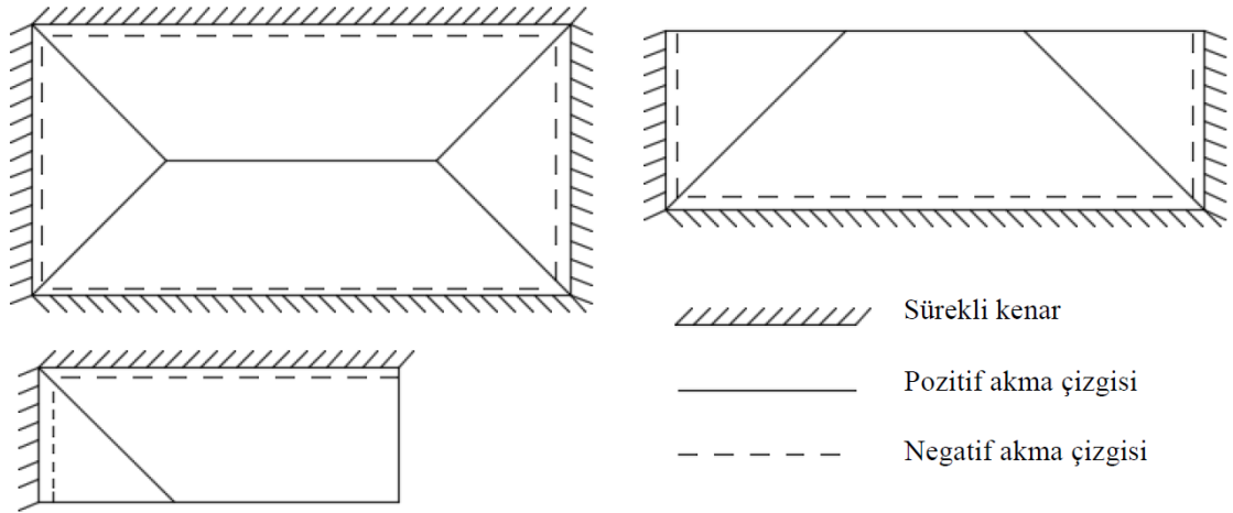
Şekil 3.7. Akma çizgileri.
